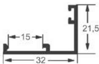
BX 026 Perfil baguetão para vidro fixo
