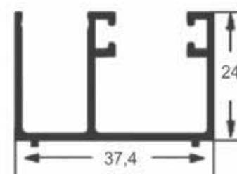
MWA 020 Trilho inferior
